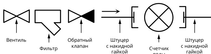
Рис. 2. Схема установки счетчика воды
